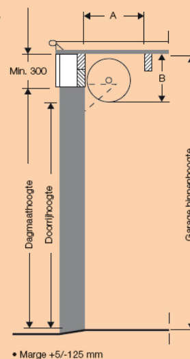
Verticale doorsnede
