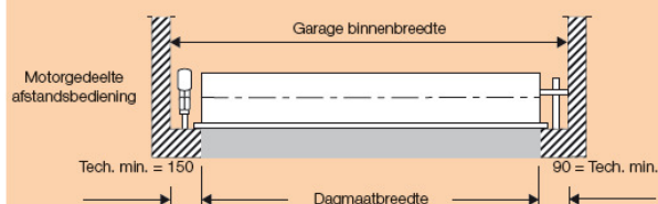
Horizontale doorsnee met en zonder afstandsbediening
